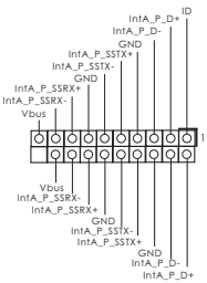
USB32_7_8
