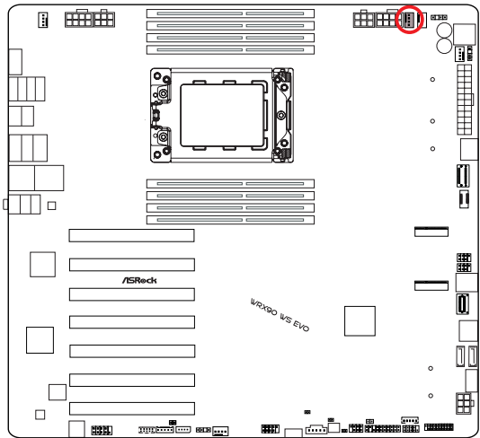
CPU_FAN1
