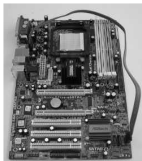
Connectez le câble de données SATA au connecteur SATAII rouge (eSATAII_BOTTOM)
