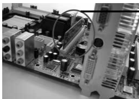
Scheda PCIE Switch nell'alloggio PCIE2/ PCIE SWITCH
