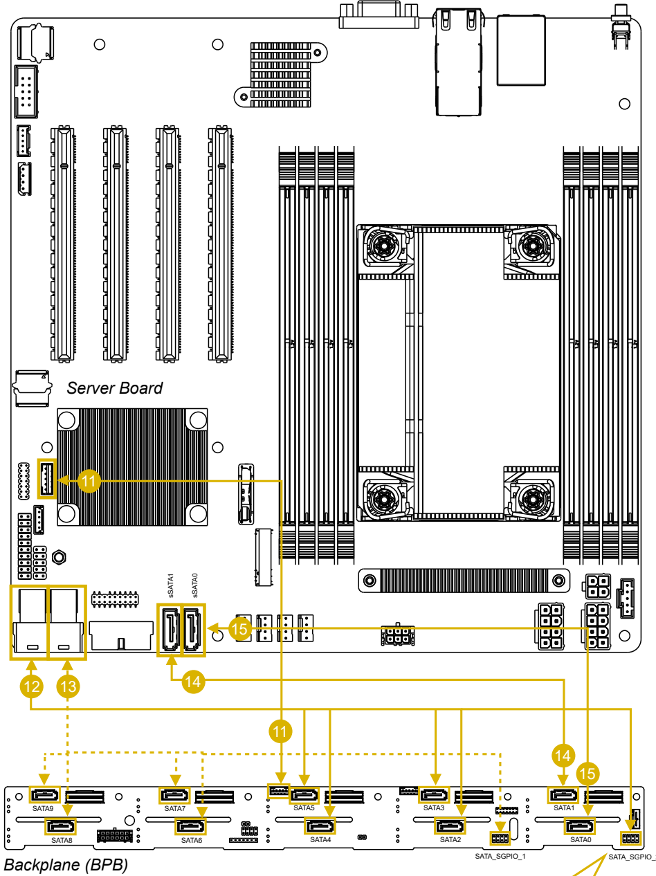
Backplane (BPB)
