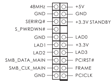
30 : TPM Header
