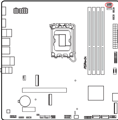
CPU_FAN1
