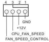
CPU_FAN1
